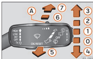
Fig. 49 Manejo del limpiaparabrisas y limpiapuneta.
